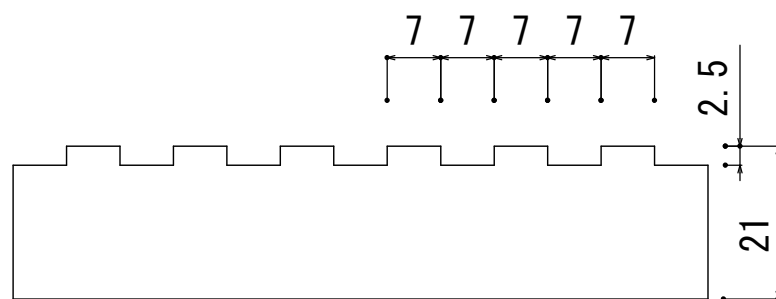
Y断面詳細図
